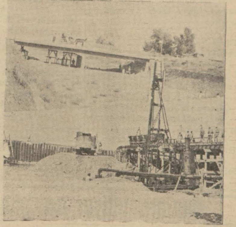
Yukarıda: Açılan kanallardan biri ve üzerindeki köprü, aşağıda Seyhanın son kısm sularını tahliye eden makine. lardan biri çalışırken
